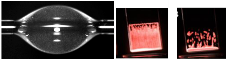
FIGURE 1 – À gauche, goutte contenant des particules fluorescente de 1\ \mu\text{m} sur une fibre en verre de 250\ \mu\text{m} de diamètre. La courbure de la fibre et ses propriétés thermiques influencent l'évaporation de la goutte. Au centre et à droite, déposition et drainage de gouttes d'émulsions sur une plaque de verre : les gouttes s'aggrègent par capillarité.
